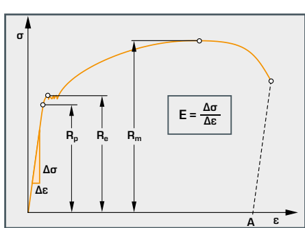
Análisis de los datos en un diagrama de tensión/alargamiento, cálculo de la resistencia
