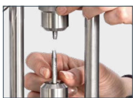
Extraer la probeta de tracción y eliminarla
