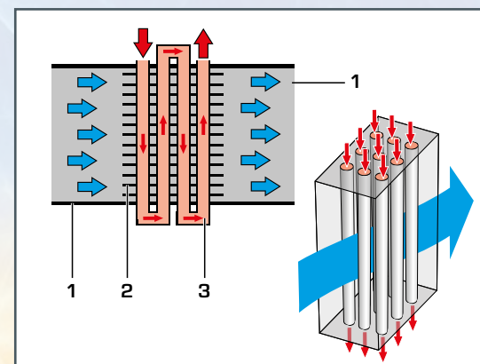
1 canal de aire, 2 aletas, 3 sección de tubo que transporta agua, ■ aire frío, ■ sección de tubo con agua caliente
