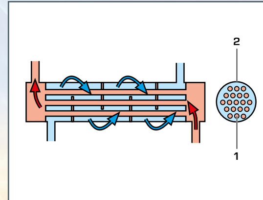
1 tubo central, 2 tubo envolvente ■ lado de agua fría, ■ lado de agua caliente
