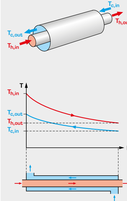
Perfiles de temperatura en un funcionamiento con flujo a contracorriente de un cambiador de calor de tubos concéntricos
