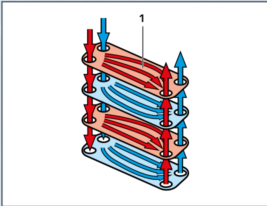
1 placa con perfil estampado ■ lado de agua fría, ■ lado de agua caliente
