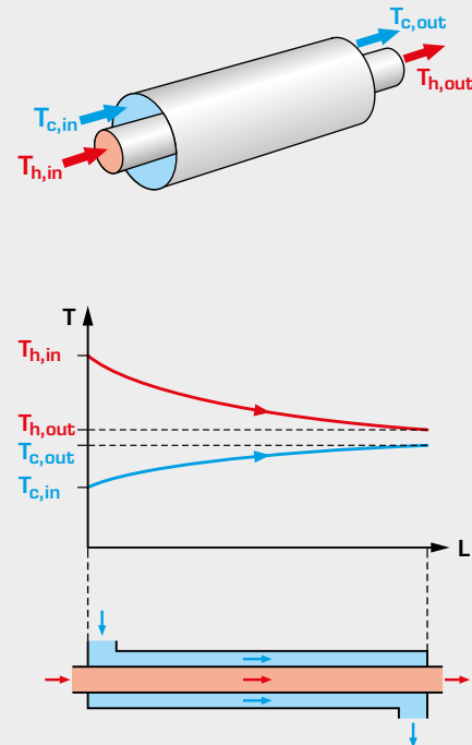
Perfiles de temperatura en un funcionamiento con flujo paralelo de un cambiador de calor de tubos concéntricos
