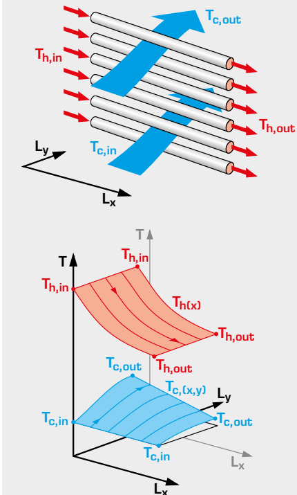
Perfil de temperatura en un solo banco de tubos con flujo cruzado mezclado transversalmente en un solo lado
